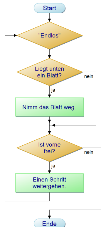
while-Schleife mit break und continue
